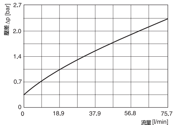
CM3 ( \Delta p/Q -特性曲線)
