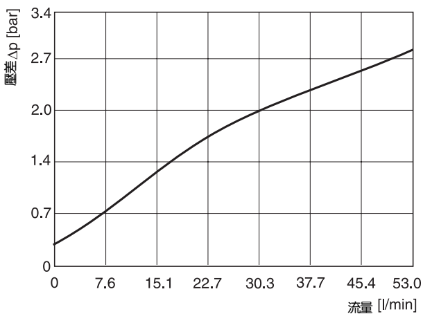
CM2 ( \Delta p/Q -特性曲線)
