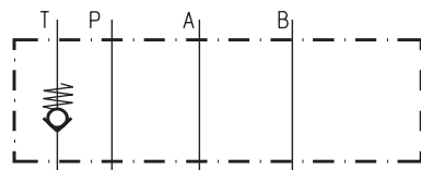
HROT 背壓或防止油壓流入
