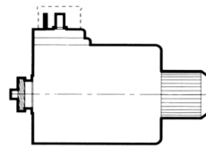
帶有插頭板 代號W
