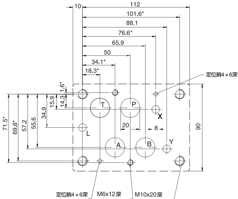
公稱尺寸 16: 連接底板 DIN 24340-A16
