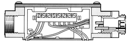
帶有 Brad Harrison 插頭外殼 代號: C 和 6
