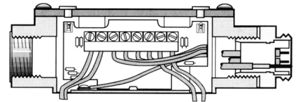
帶有顯示燈和 Brad Harrison 插頭外殼 代號: 5 和 6
