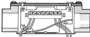
帶有顯示燈和接線端子 代號: C 和 5
