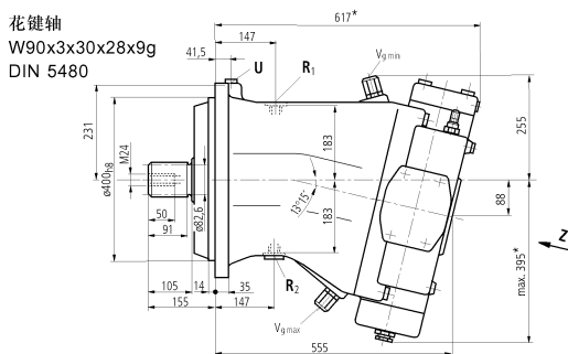
Y向视图
